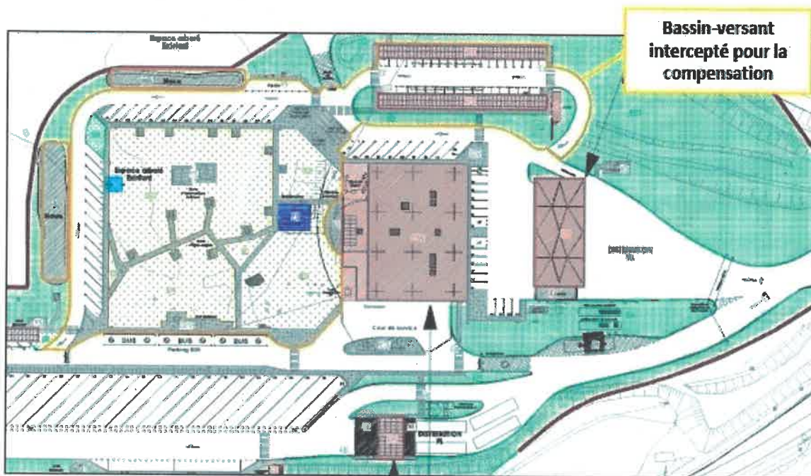
Figure 6 : Présentation du bassin versant intercepté pour l'ouvrage de compensation EP
