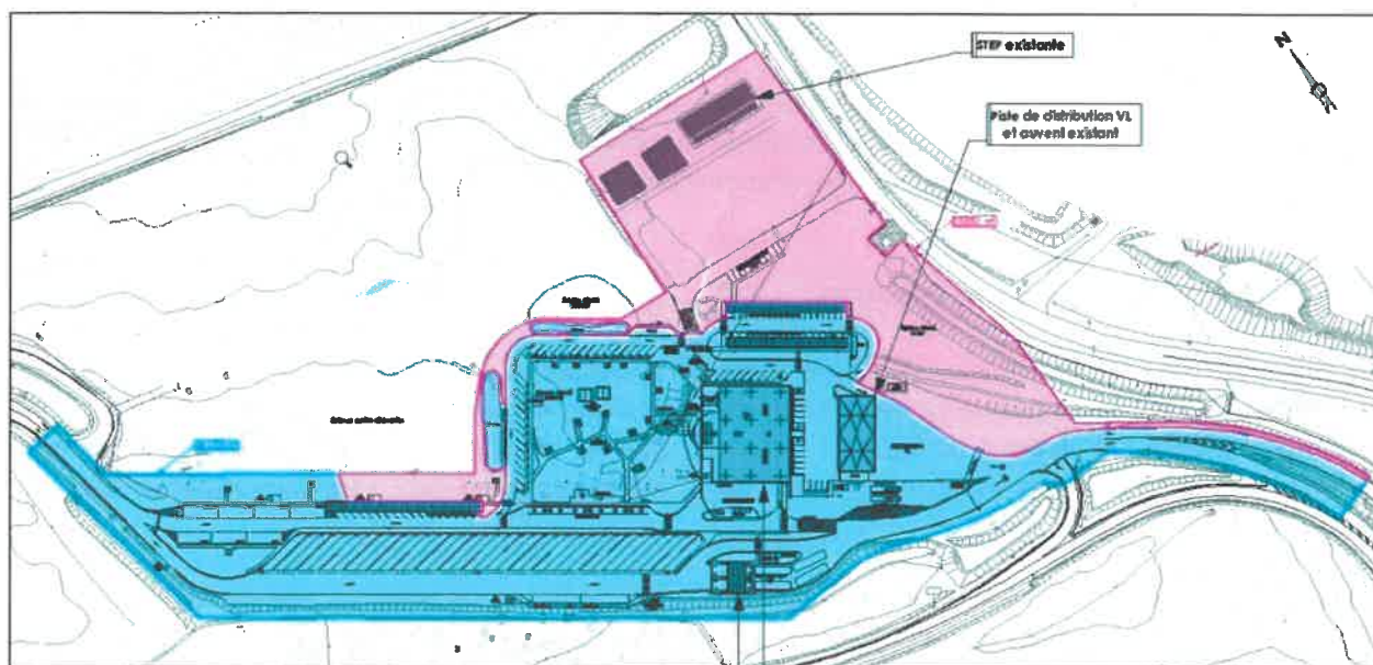
Figure 5 : Découpage en bassins versants de l'aire de service des Palombières
