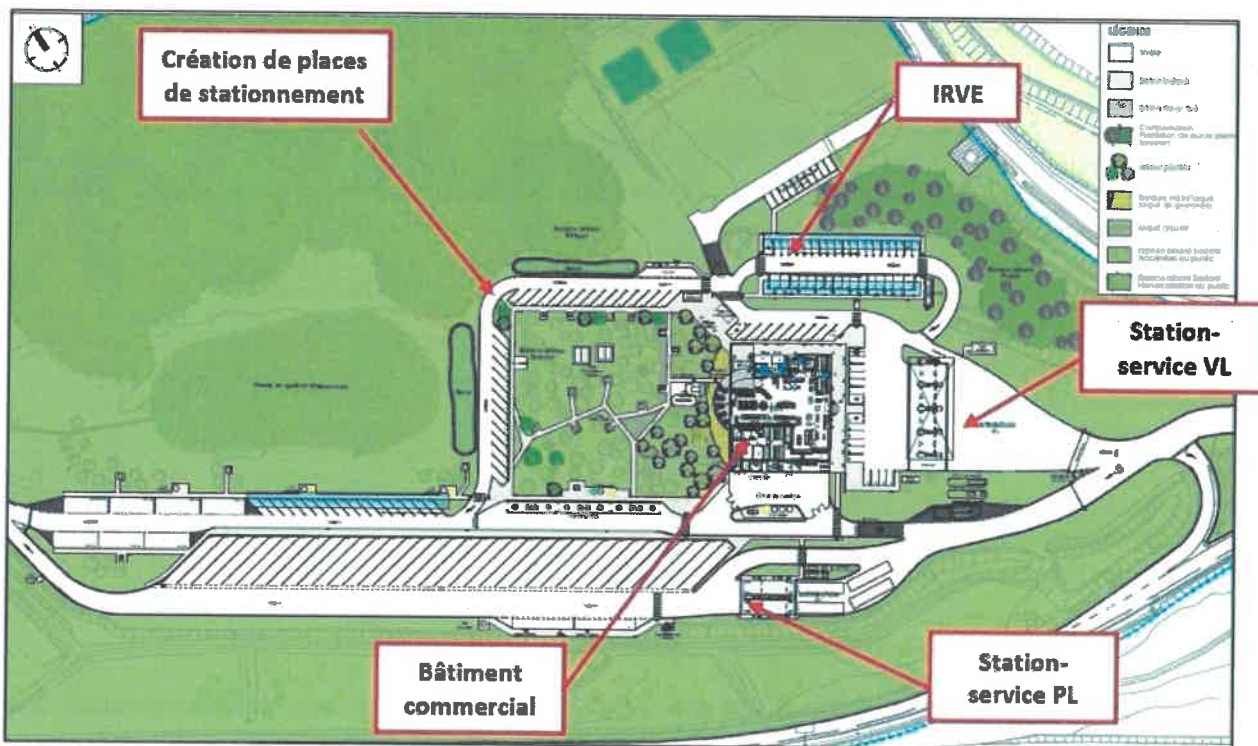
Figure 3 : Plan de masse du projet de réaménagement de l'aire des Palombières
